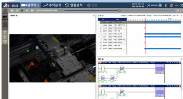
[녹화영상/Ladder/Gantt Chart 기반 운영재현]
